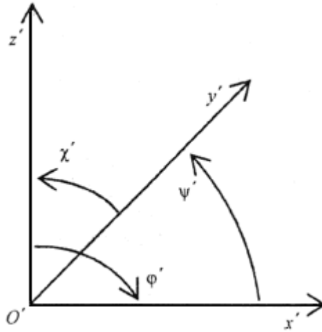
Рисунок Б.1 - Степени свободы фундамента
